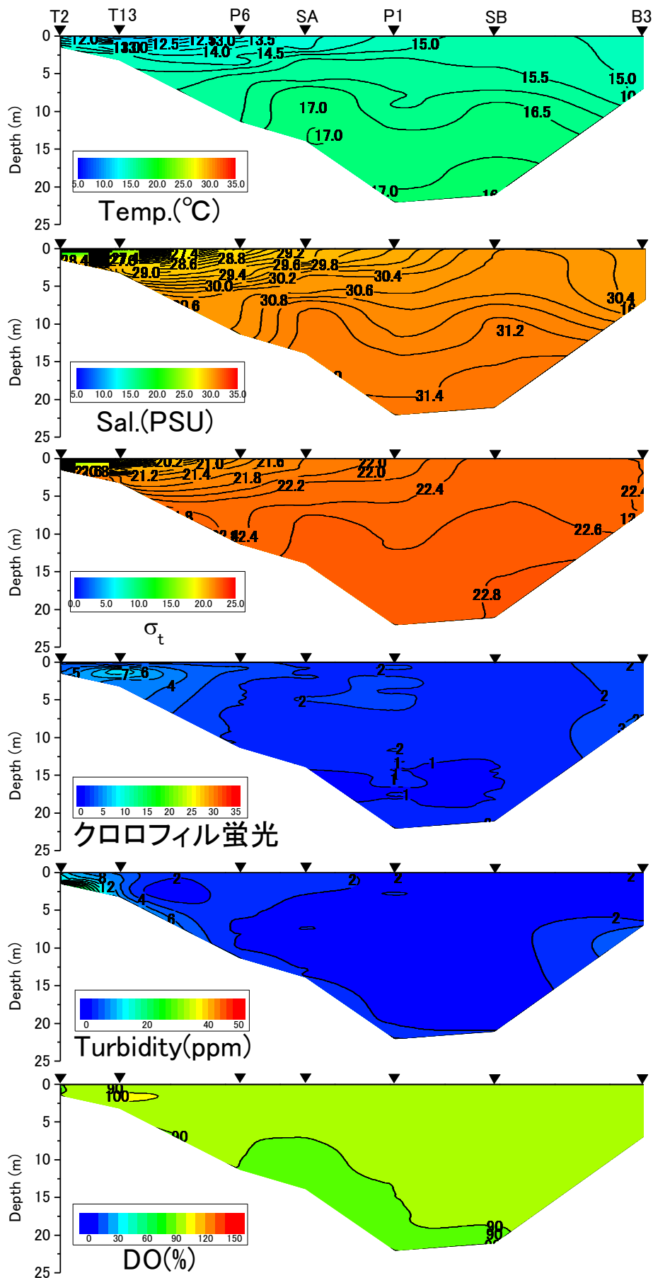
2019年12月4日における水温、塩分、密度 \sigma_t 、クロロフィル蛍光値、濁度、DO飽和度 (定点SCは欠測)
