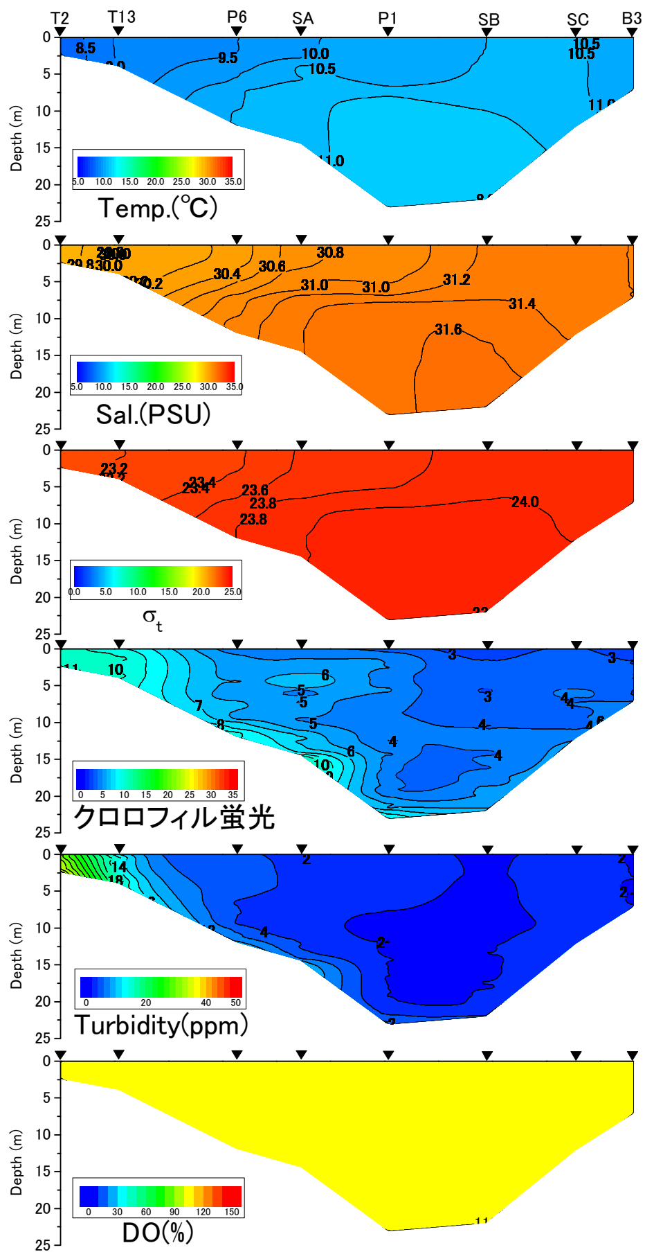
2019年1月28日にける水温、塩分、密度 \sigma_t 、クロロフィル蛍光値、濁度、DO飽和度
