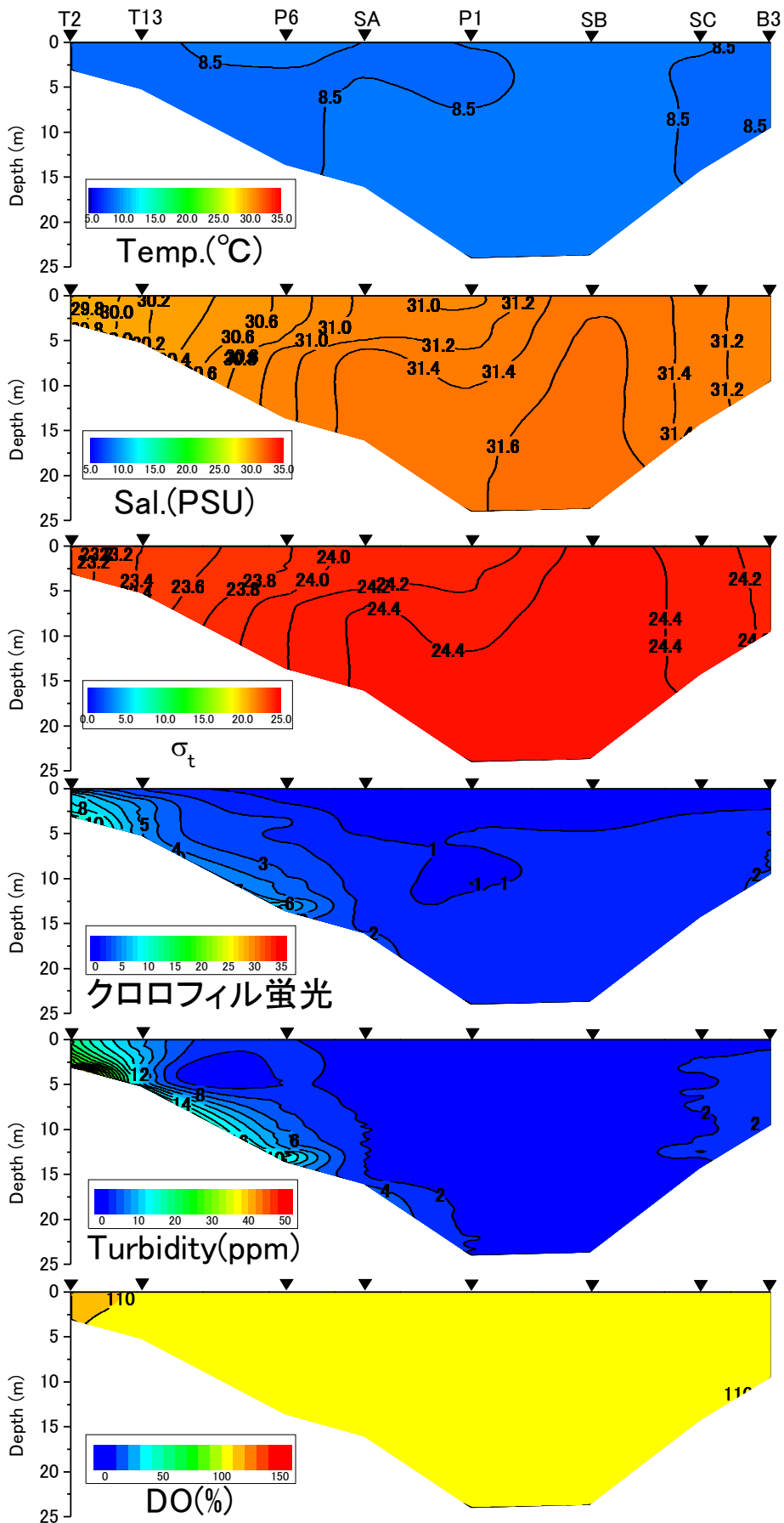
2018年2月22日における水温、塩分、密度 \sigma_t 、クロロフィル蛍光値、濁度、DO飽和度
