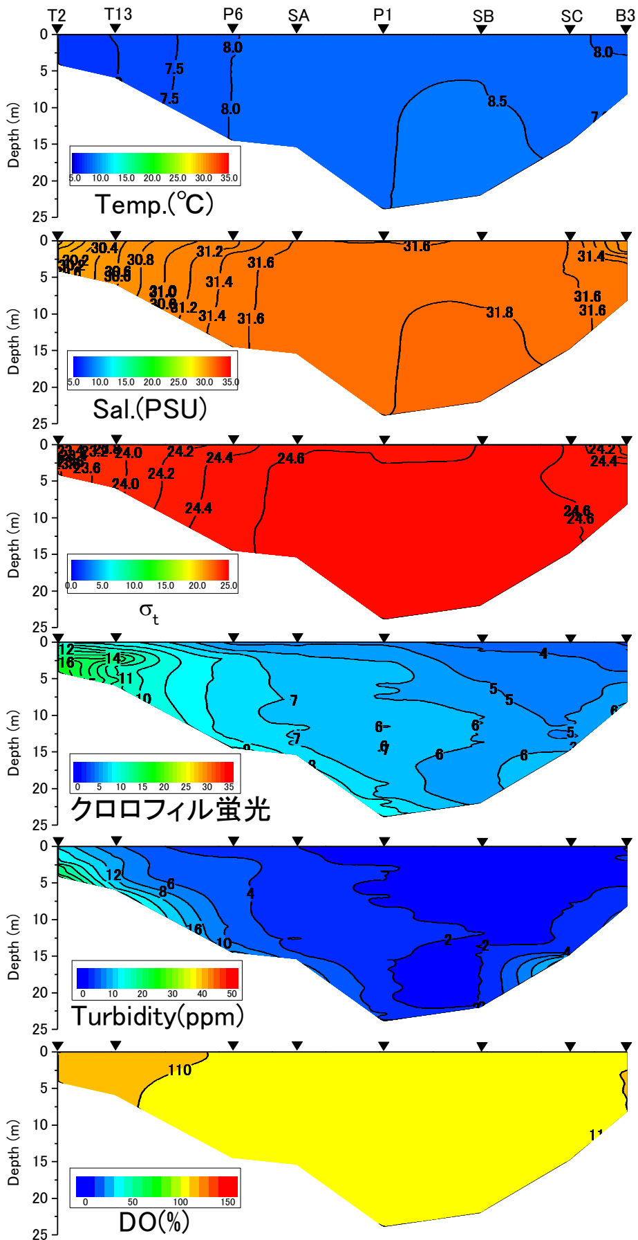
2018年2月15日における水温、塩分、密度 \sigma_t 、クロロフィル蛍光値、濁度、DO飽和度
