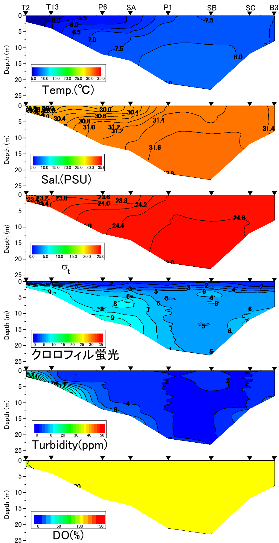
2018年2月8日における水温、塩分、密度 \sigma_t 、クロロフィル蛍光値、濁度、DO飽和度
