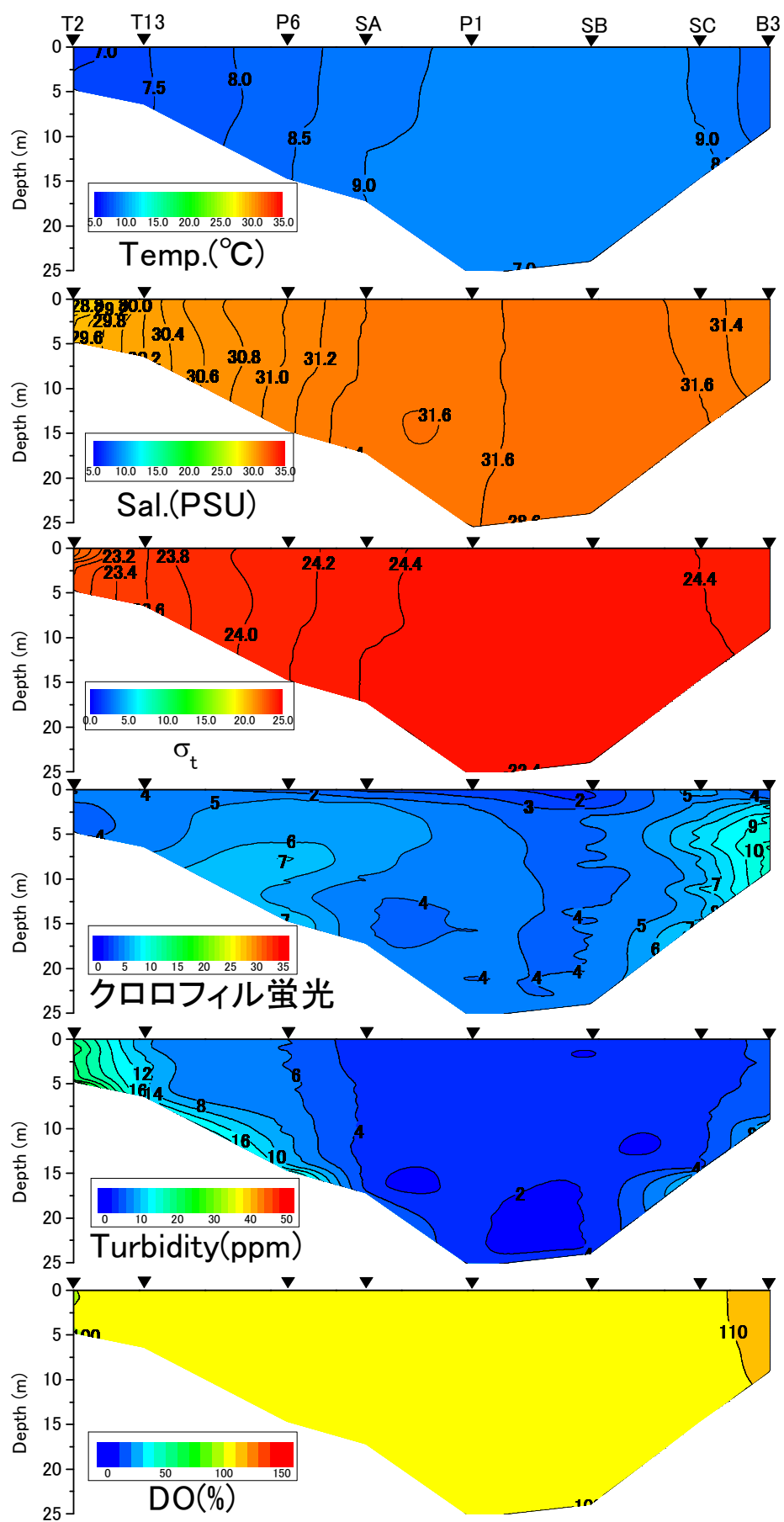
2018年2月1日における水温、塩分、密度 \sigma_t 、クロロフィル蛍光値、濁度、DO飽和度
