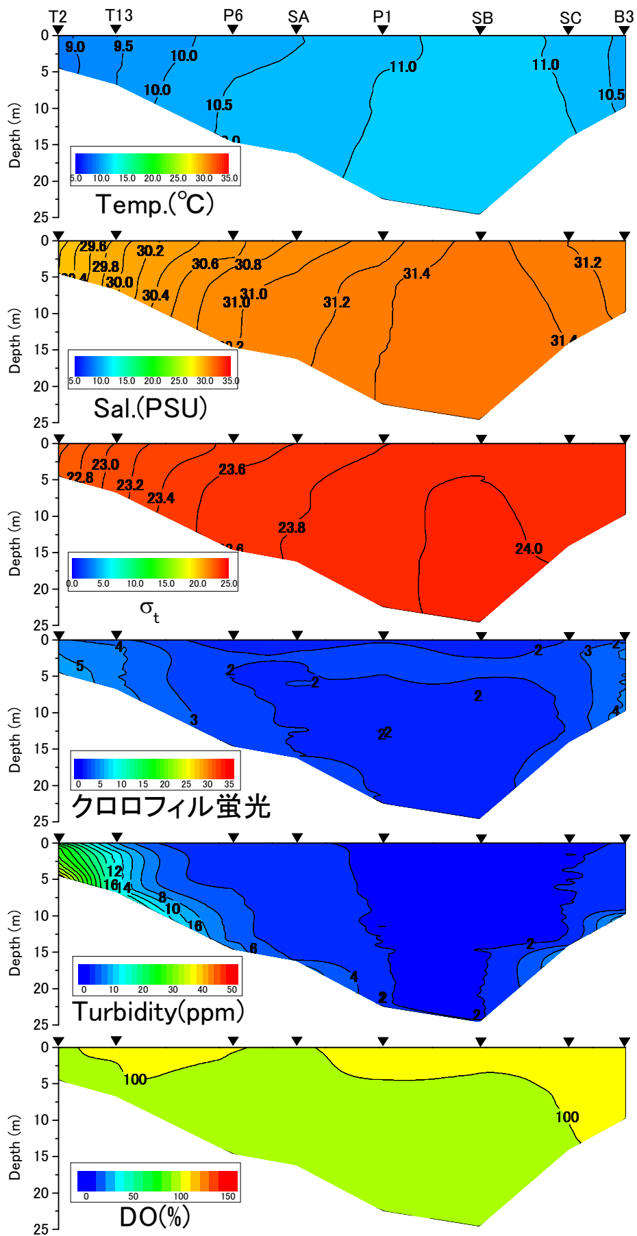
2018年1月4日における水温、塩分、密度 \sigma_t 、クロロフィル蛍光値、濁度、DO飽和度
