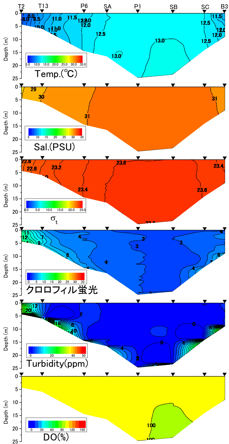
2017年12月18日における水温、塩分、密度 \sigma_t 、クロロフィル蛍光値、濁度、DO飽和度
