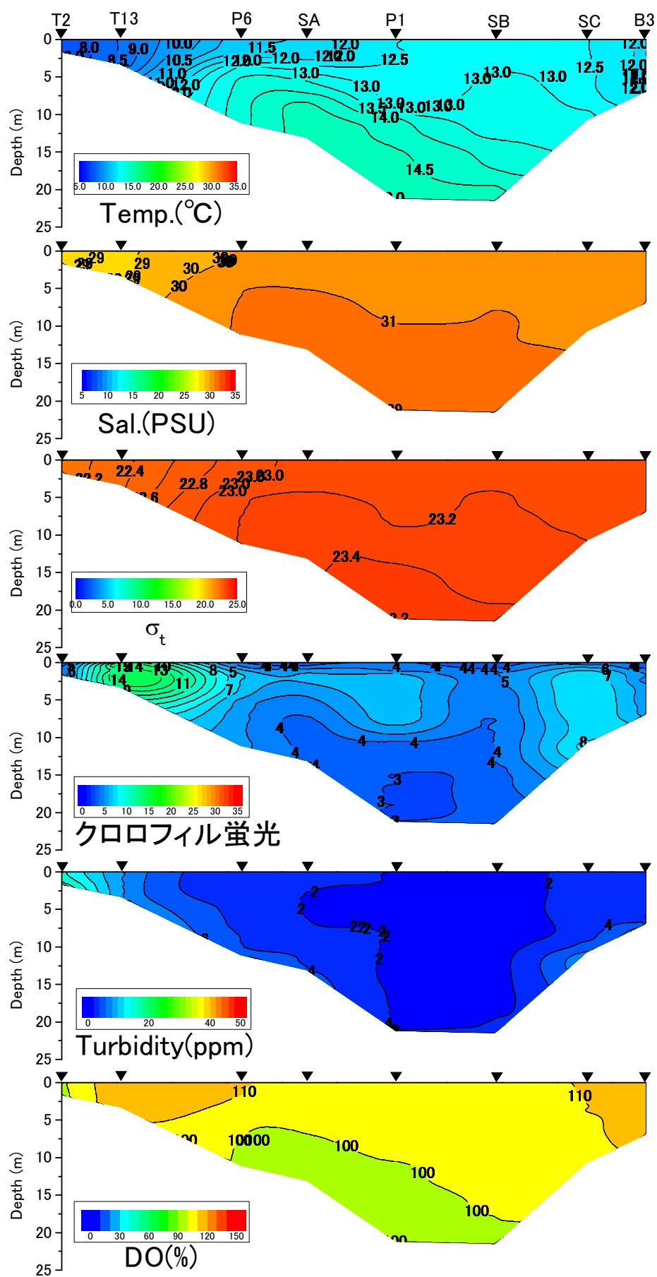
2017年12月13日における水温、塩分、密度 \sigma_t 、クロロフィル蛍光値、濁度、DO飽和度
