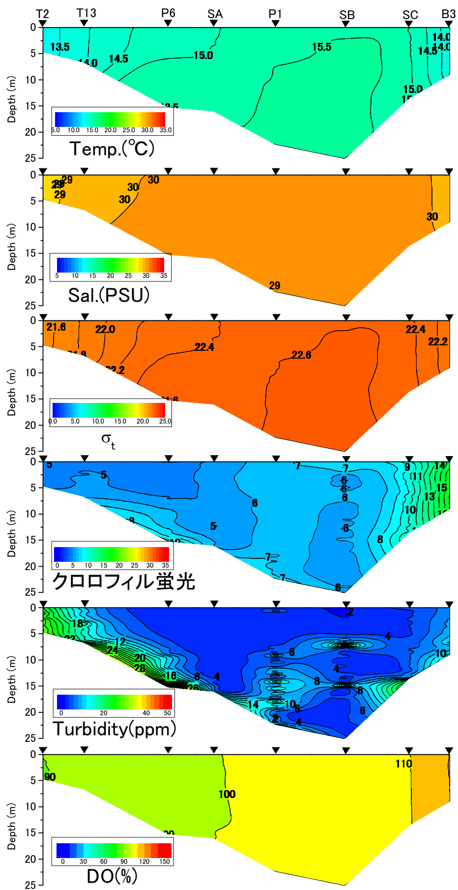
2017年12月4日における水温、塩分、密度 \sigma_t 、クロロフィル蛍光値、濁度、DO飽和度
