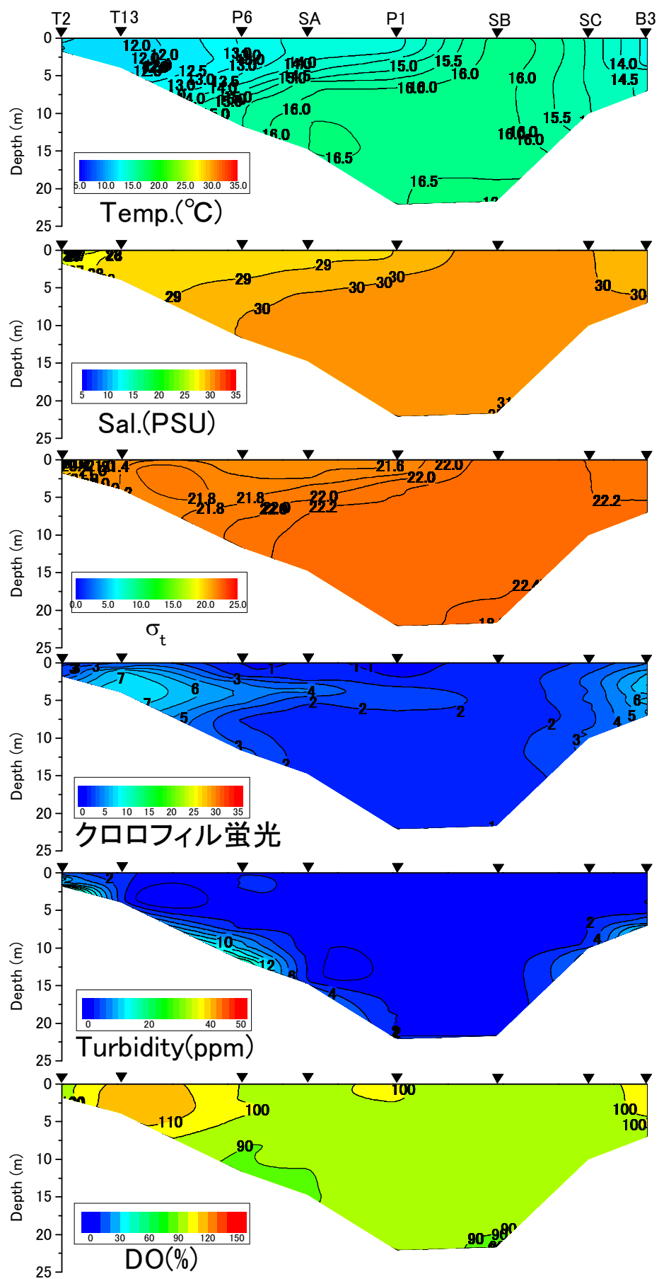
2017年11月27日における水温、塩分、密度 \sigma_t 、クロロフィル蛍光値、濁度、DO飽和度
