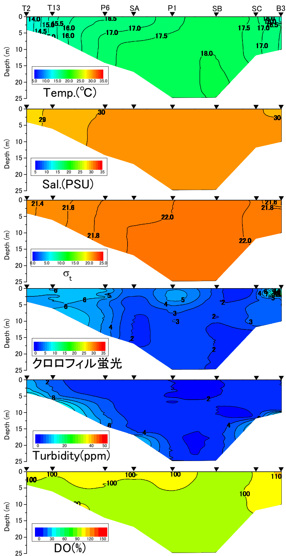
2017年11月20日における水温、塩分、密度 \sigma_t 、クロロフィル蛍光値、濁度、DO飽和度
