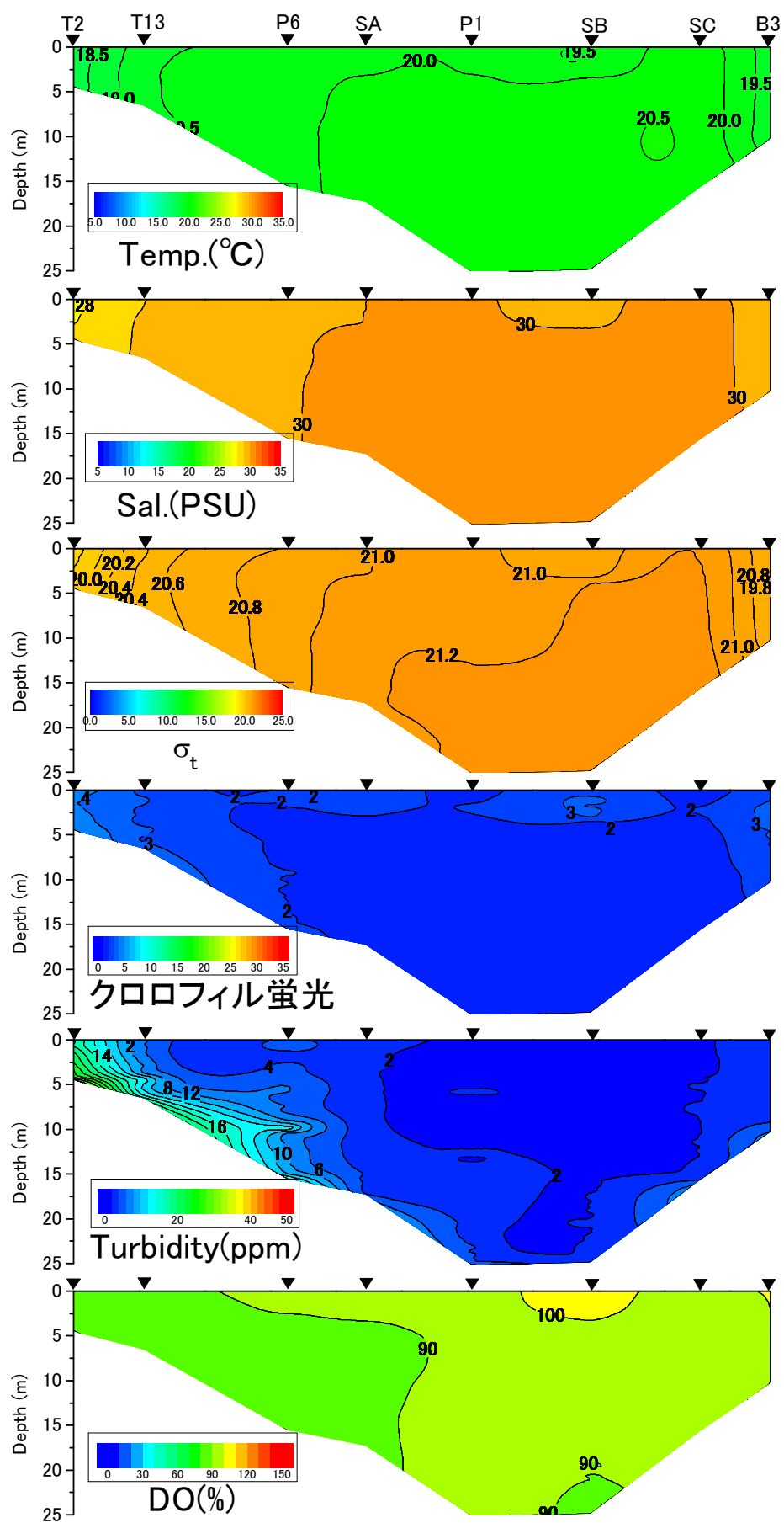
2017年11月5日における水温、塩分、密度 \sigma_t 、クロロフィル蛍光値、濁度、DO飽和度
