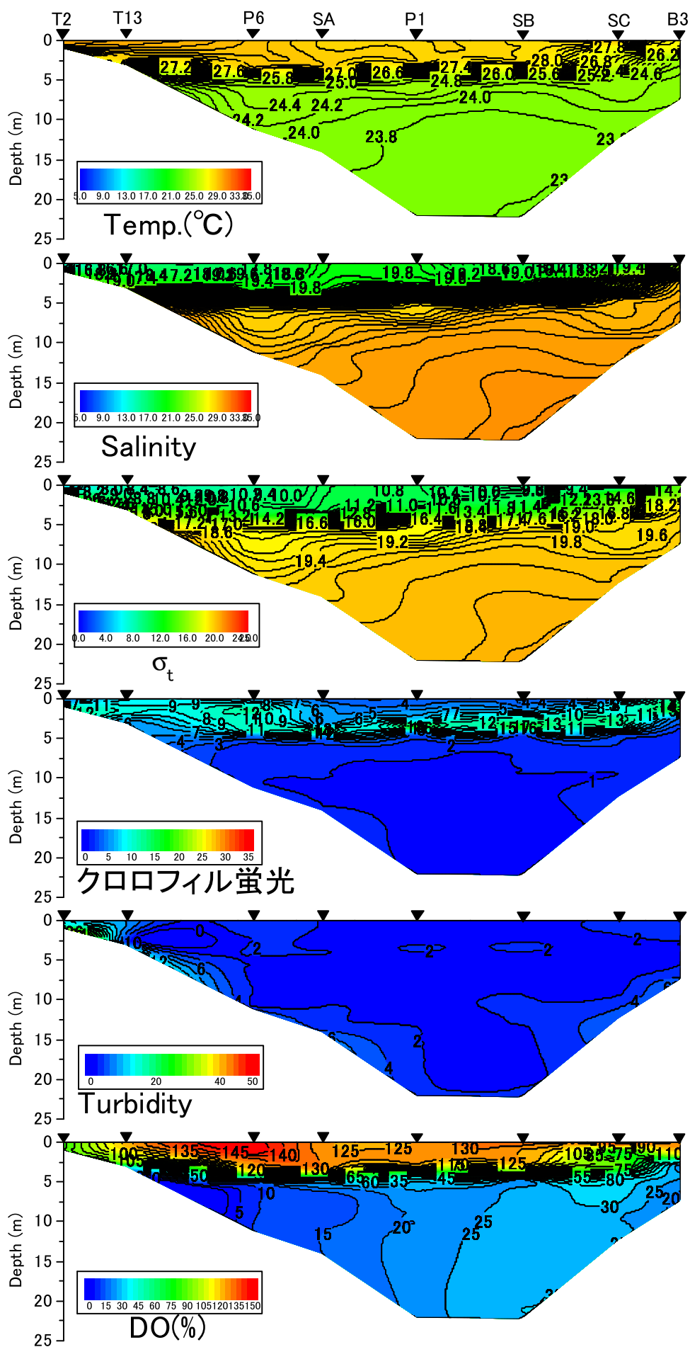
2017年7月17日における水温、塩分、密度 \sigma_t 、クロロフィル蛍光値、濁度、DO飽和度
