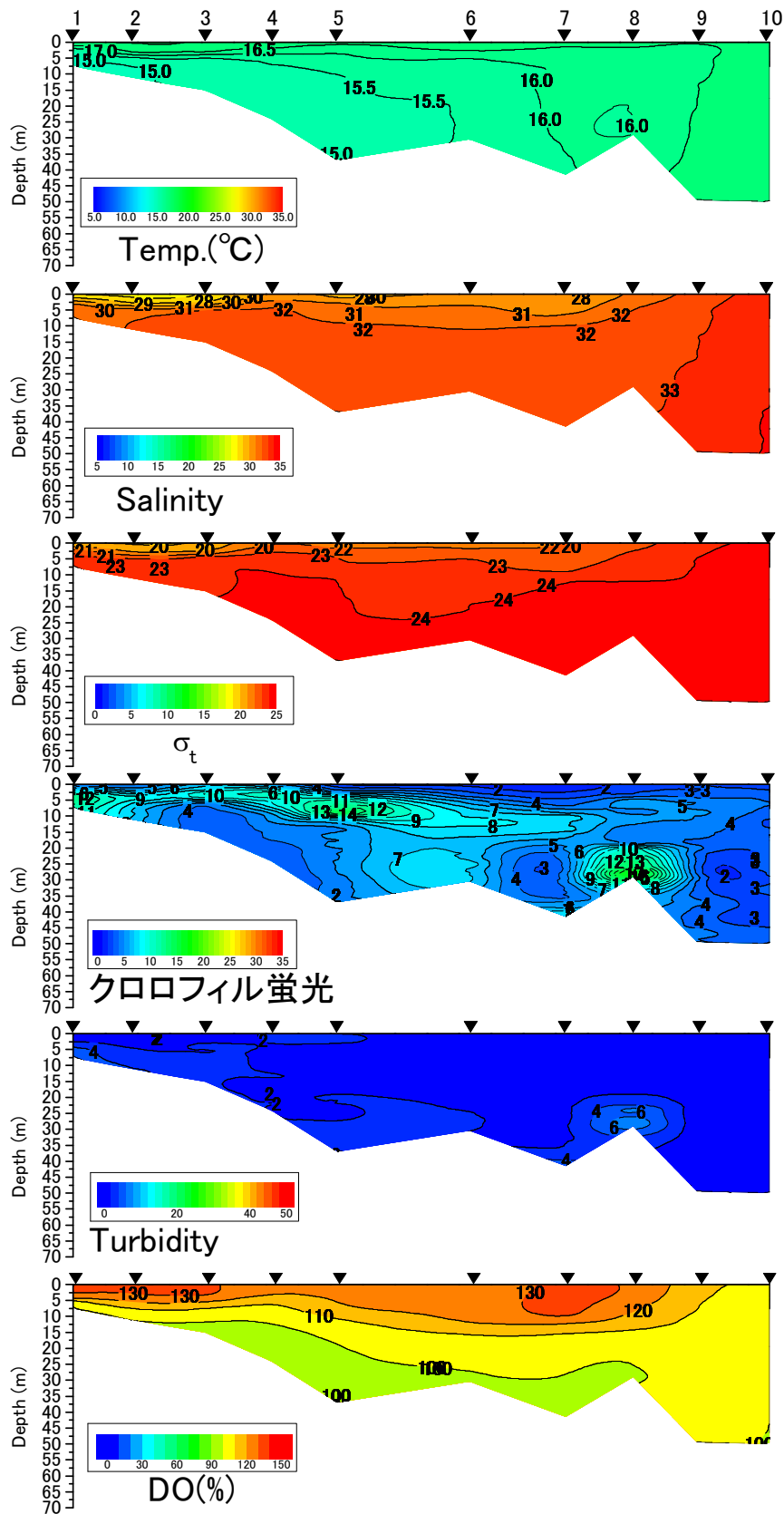
有明海中央ラインの水温(°C)、塩分、密度( \sigma_t )、クロロフィル蛍光強度、濁度、溶存酸素飽和度(DO%)の鉛直面図(国土交通省の調査による) (2017年4月25日)
