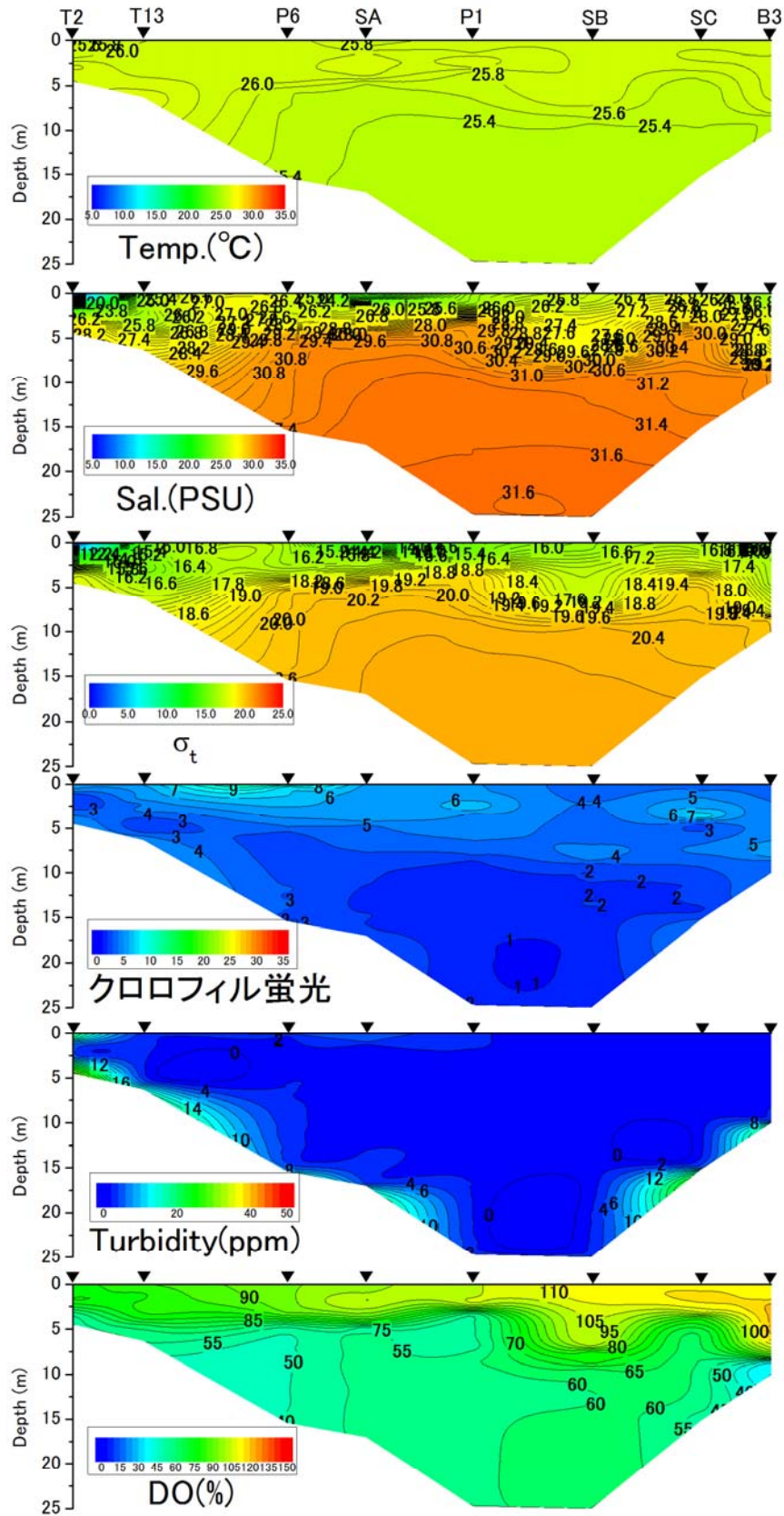
2016年9月29日における水温、塩分、密度 \sigma_t 、クロロフィル蛍光値、濁度DO飽和度の鉛直分布
