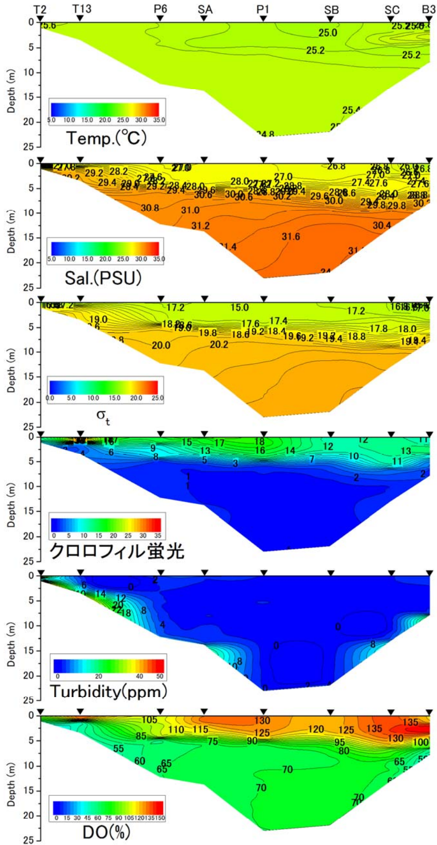
2016年9月25日における水温、塩分、密度 \sigma_t 、クロロフィル蛍光値、濁度DO飽和度の鉛直分布
