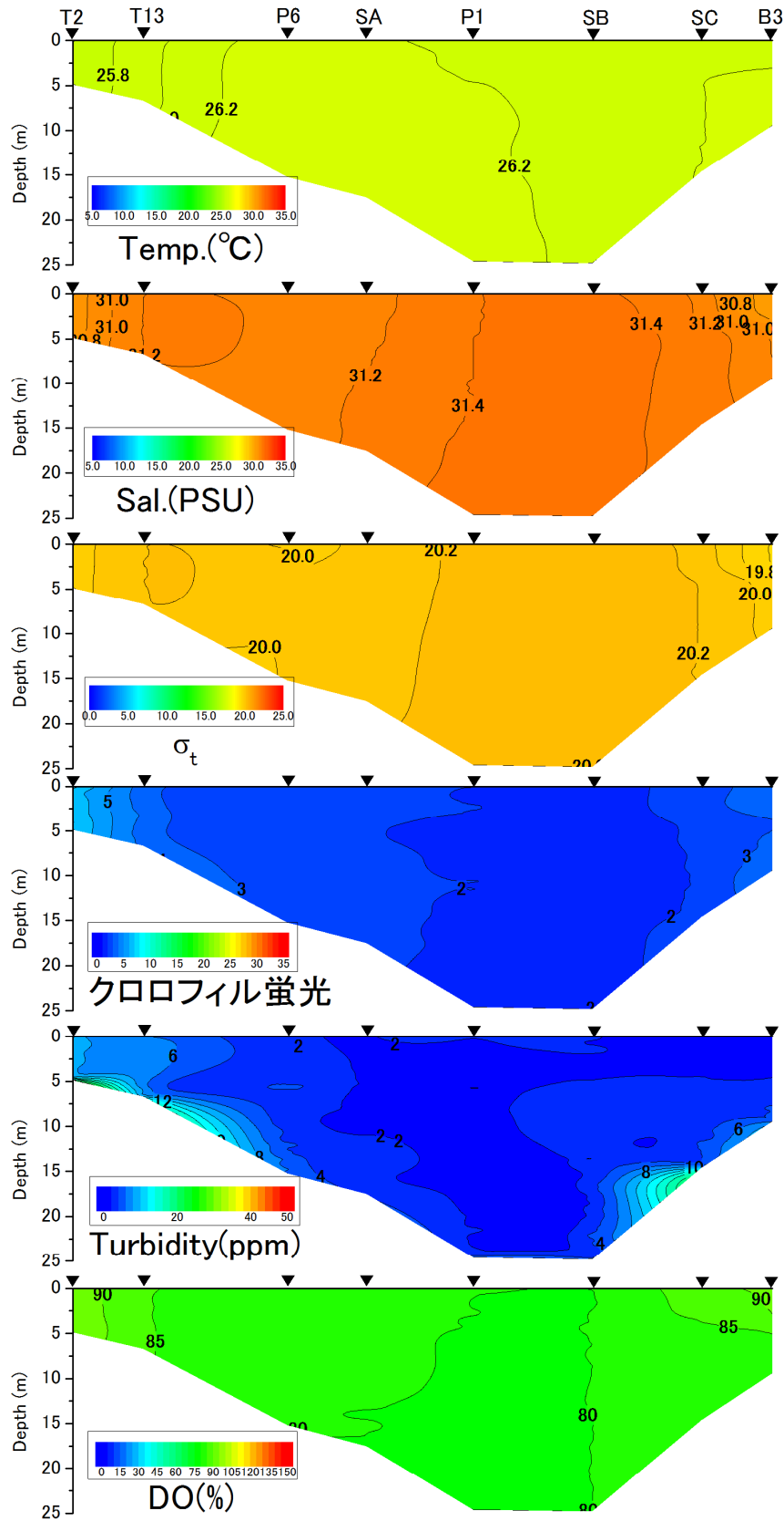
2016年9月1日における水温、塩分、密度 \sigma_t 、クロロフィル蛍光値、濁度DO飽和度の鉛直分布
