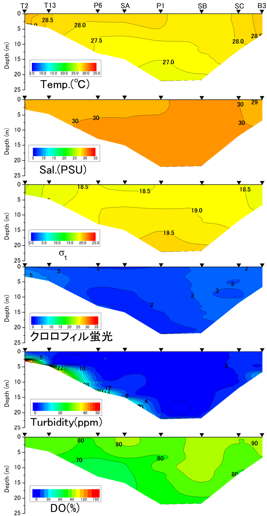
2016年8月24日における水温、塩分、密度 \sigma_t 、クロロフィル蛍光値、濁度DO飽和度の鉛直分布
