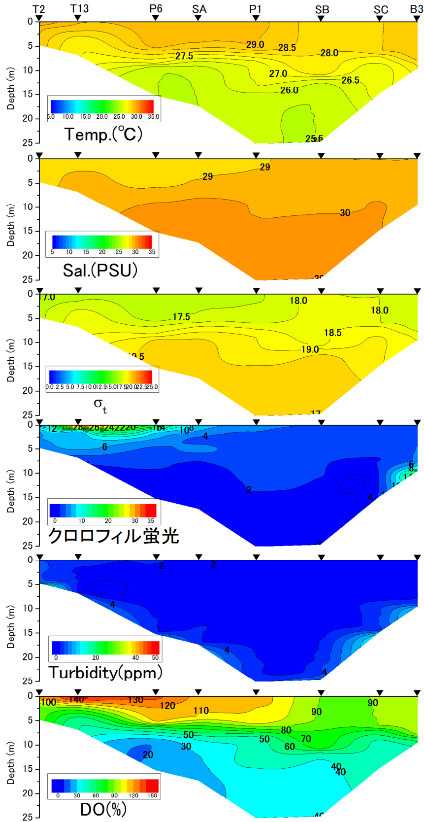
2016年8月18日における水温、塩分、密度 \sigma_t 、クロロフィル蛍光値、濁度DO飽和度の鉛直分布
