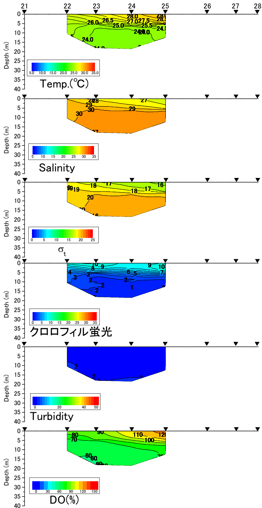
有明海東ラインの水温(°C)、塩分、密度( \sigma_t )、クロロフィル蛍光強度、濁度、溶存酸素飽和度(DO%)の鉛直面図(国土交通省の調査による) (2016年8月3日)
