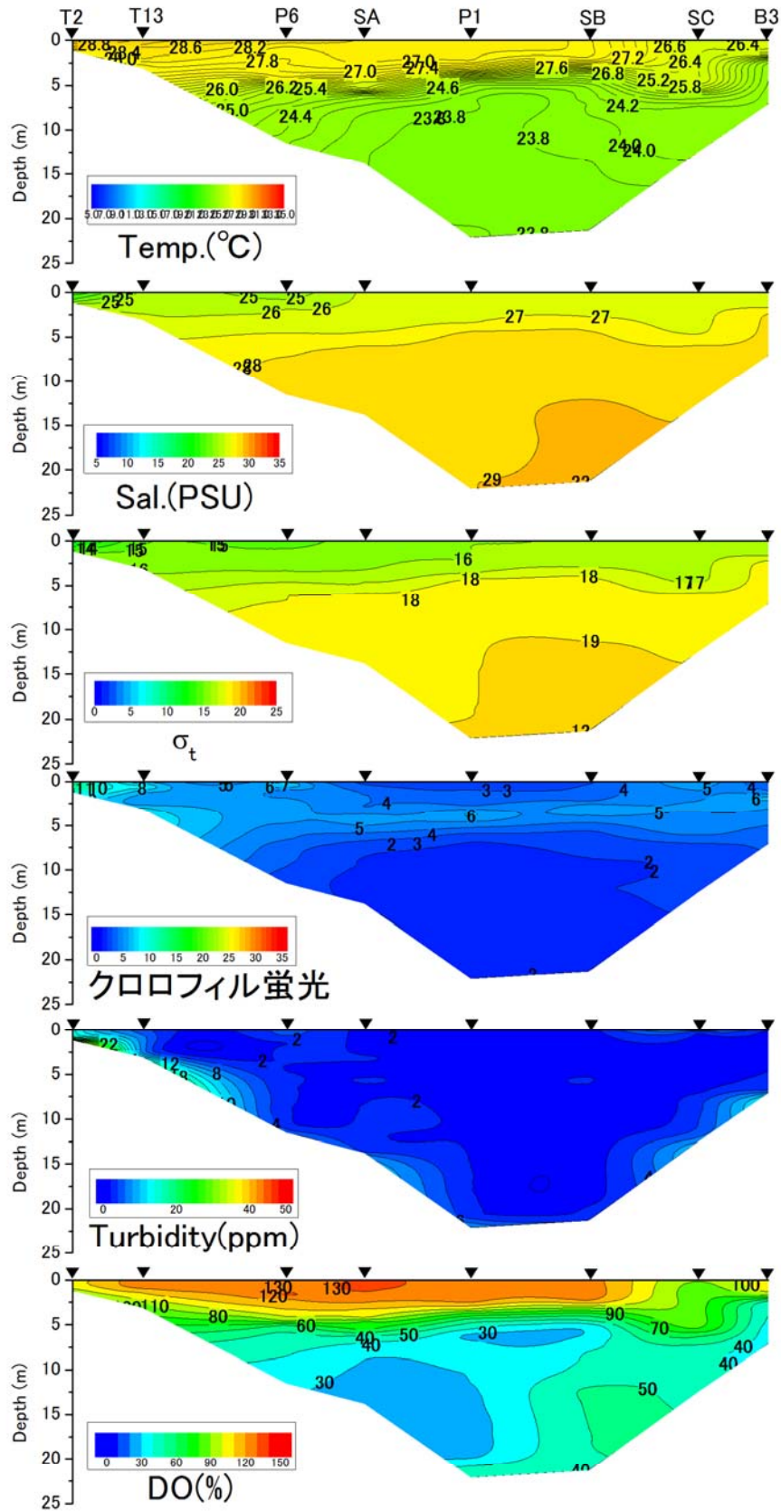
2016年7月27日における水温、塩分、密度 \sigma_t 、クロロフィル蛍光値、濁度DO飽和度の鉛直分布
