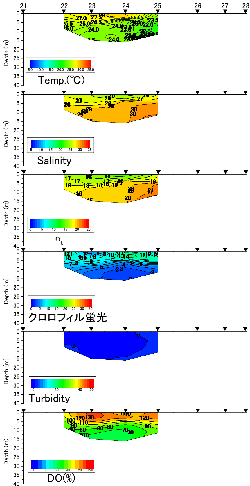
有明海東ラインの水温(°C)、塩分、密度( \sigma_t )、クロロフィル蛍光強度、濁度、溶存酸素飽和度(DO%)の鉛直面図(国土交通省の調査による) (2016年7月26日)
