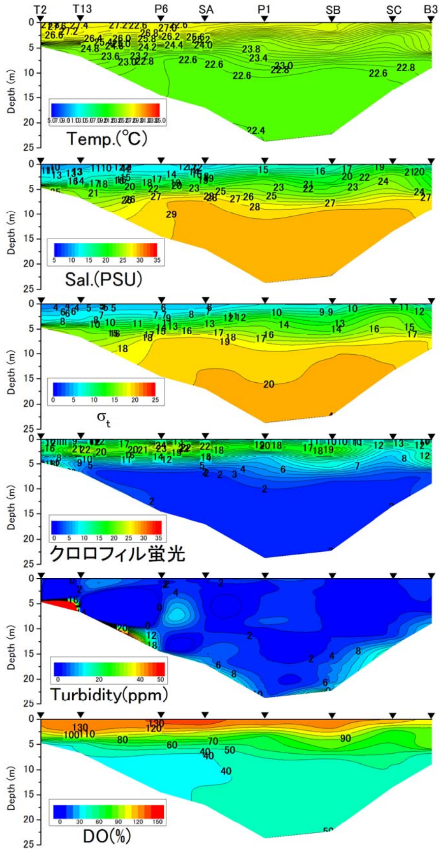
2016年7月5日における水温、塩分、密度 \sigma_t 、クロロフィル蛍光値、濁度DO飽和度の鉛直分布
