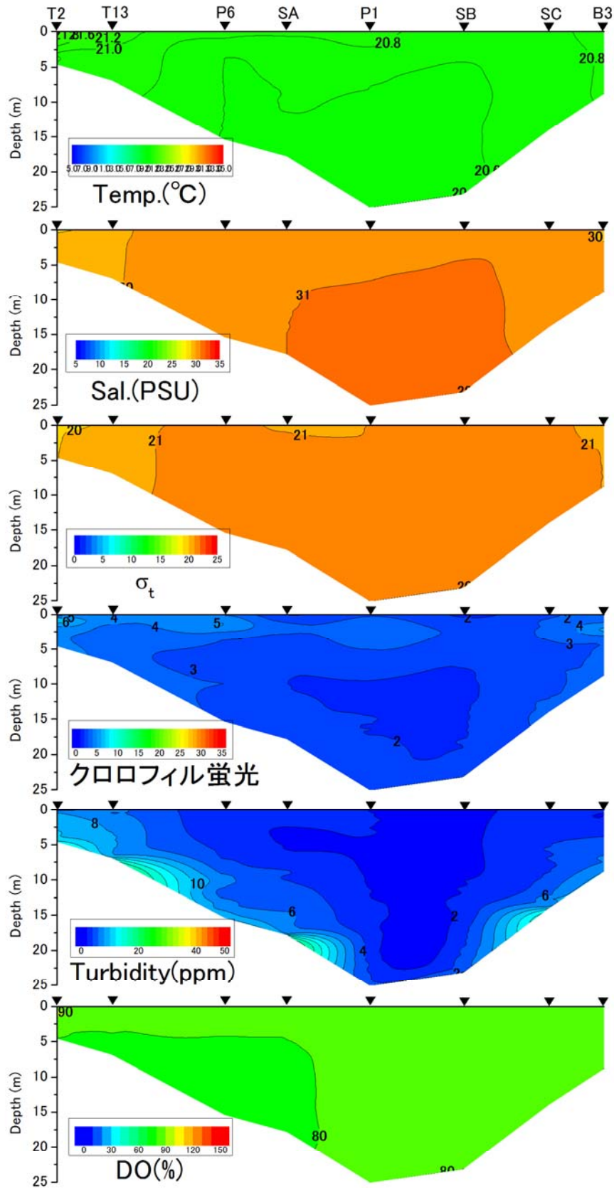
2016年6月6日における水温、塩分、密度 \sigma_t 、クロロフィル蛍光値、濁度DO飽和度の鉛直分布
