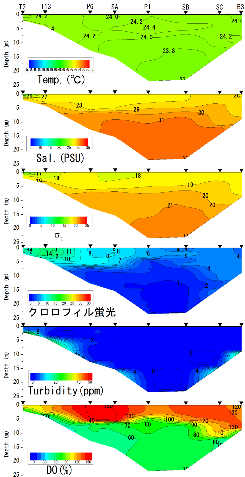
2015年9月24日における水温、塩分、密度 \sigma_t 、クロロフィル蛍光値、濁度DO飽和度の鉛直分布
