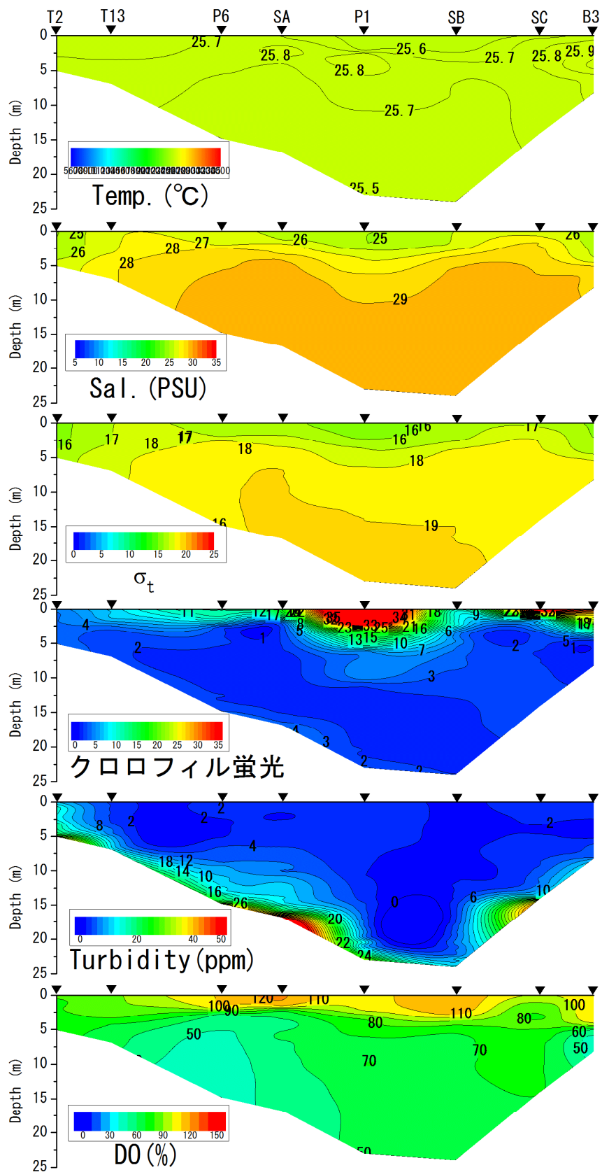
2015年8月31日における水温、塩分、密度 \sigma_t 、クロロフィル蛍光値、濁度DO飽和度の鉛直分布
