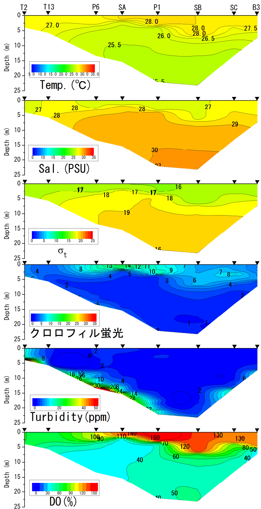
2015年8月17日における水温、塩分、密度 \sigma_t 、クロロフィル蛍光値、濁度DO飽和度の鉛直分布
