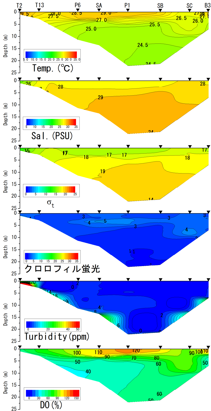
2015年8月6日における水温、塩分、密度 \sigma_t 、クロロフィル蛍光値、濁度DO飽和度の鉛直分布
