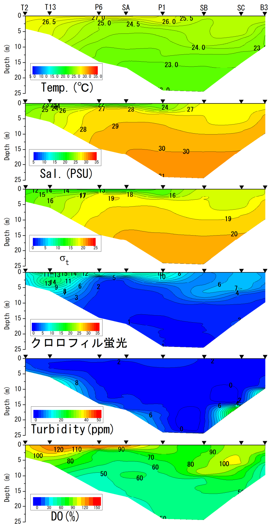
2015年7月29日における水温、塩分、密度 \sigma_t 、クロロフィル蛍光値、濁度DO飽和度の鉛直分布
