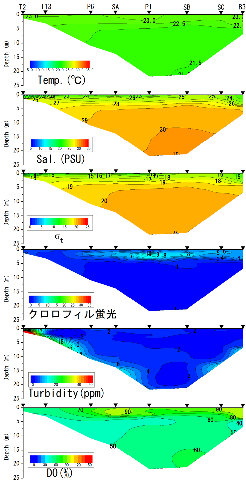
2015年7月8日における水温、塩分、密度 \sigma_t 、クロロフィル蛍光値、濁度DO飽和度の鉛直分布
