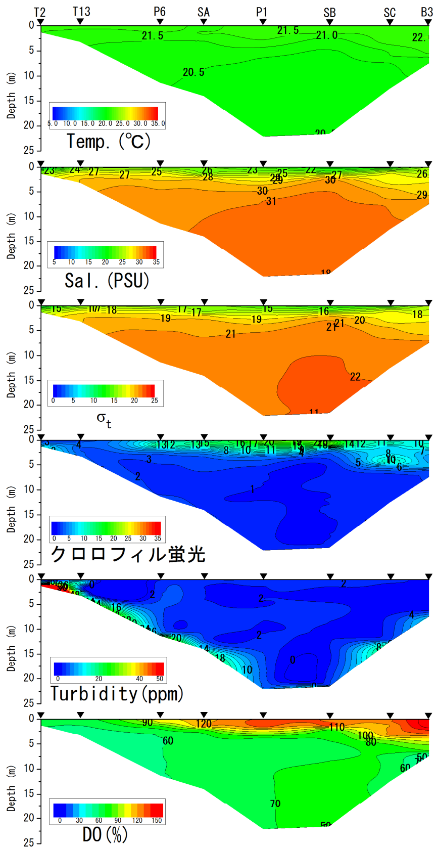
2015年6月10日における水温、塩分、密度 \sigma_t 、クロロフィル蛍光値、濁度DO飽和度の鉛直分布
