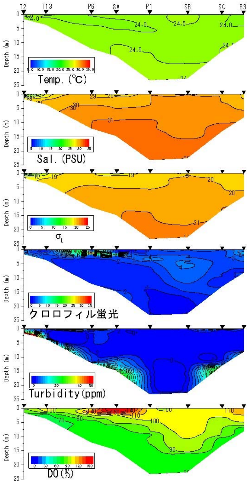
2014年10月3日における水温、塩分、密度 \sigma_t 、クロロフィル蛍光値、濁度、DO飽和度
