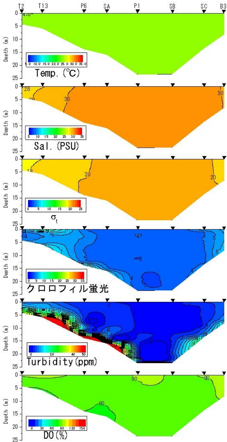
2014年9月26日における水温、塩分、密度 \sigma_t 、クロロフィル蛍光値、濁度、DO飽和度
