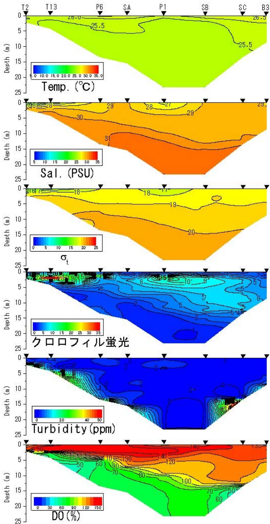
2014年9月17日における水温、塩分、密度 \sigma_t 、クロロフィル蛍光値、濁度、DO飽和度
