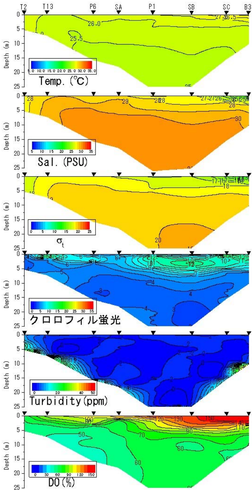
2014年9月10日における水温、塩分、密度 \sigma_t 、クロロフィル蛍光値、濁度、DO飽和度
