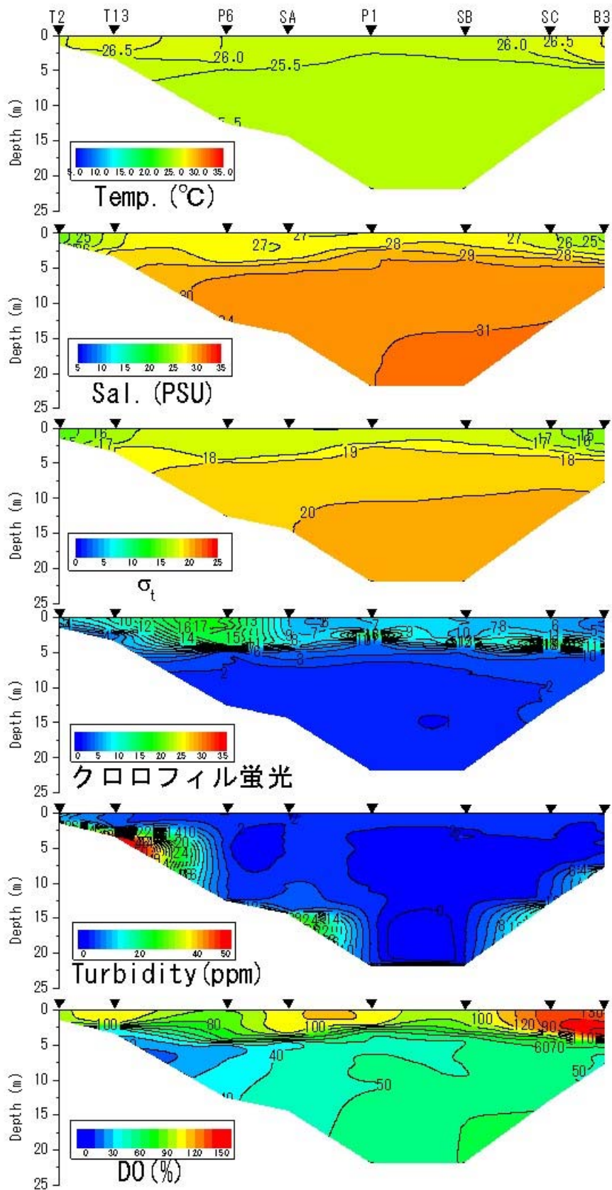
2014年9月3日における水温、塩分、密度 \sigma_t 、クロロフィル蛍光値、濁度、DO飽和度
