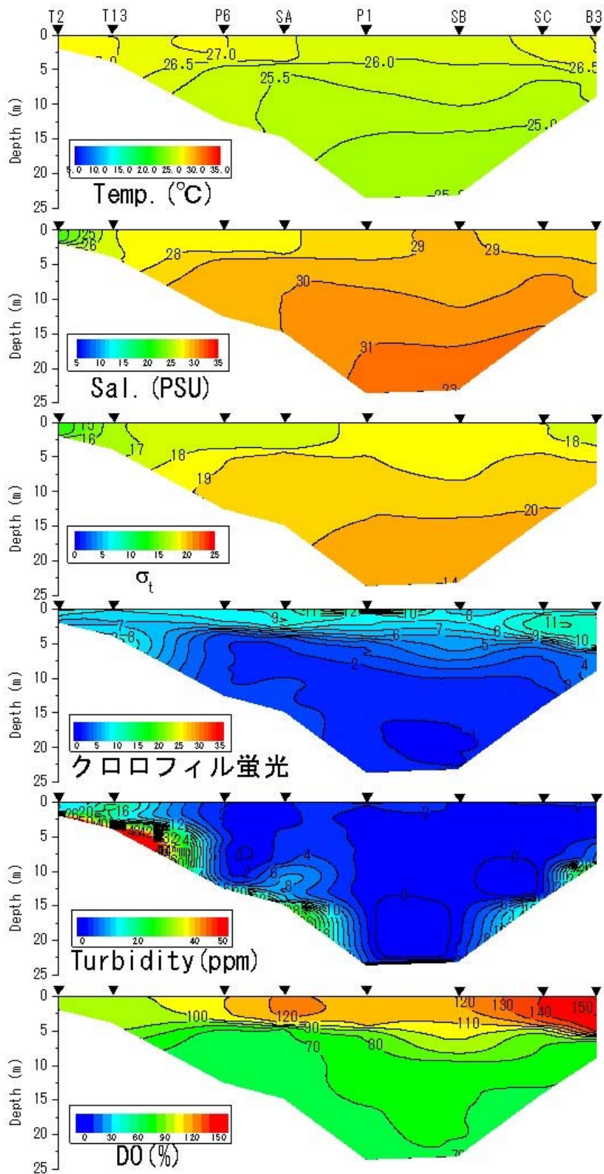
2014年8月18日における水温、塩分、密度 \sigma_t 、クロロフィル蛍光値、濁度、DO飽和度
