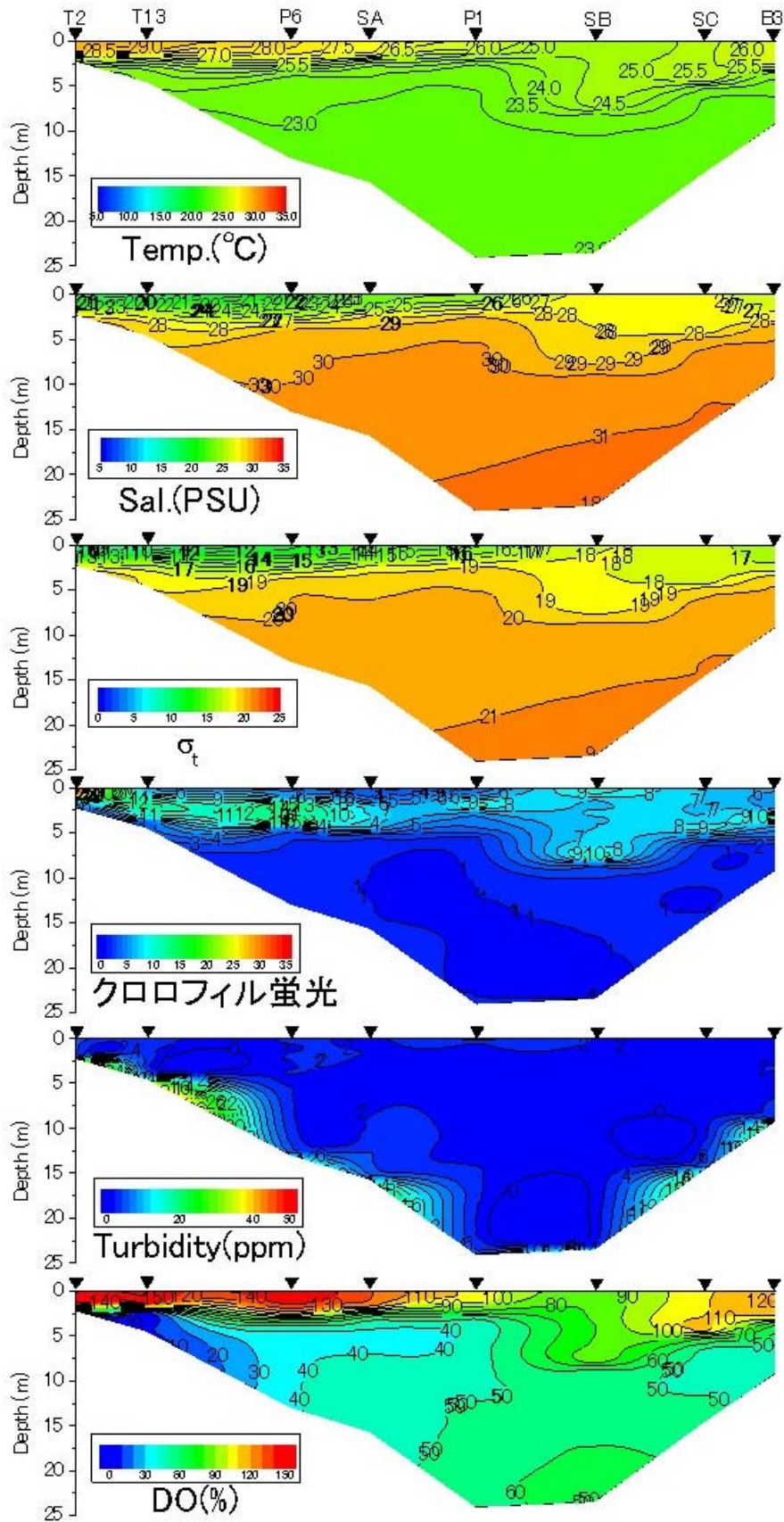
2014年7月22日における水温、塩分、密度 \sigma_t 、クロロフィル蛍光値、濁度、DO飽和度
