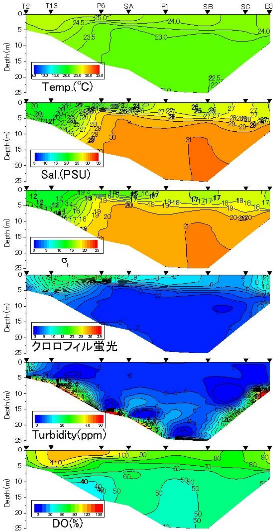
2014年7月13日における水温、塩分、密度 \sigma_t 、クロロフィル蛍光値、濁度、DO飽和度
