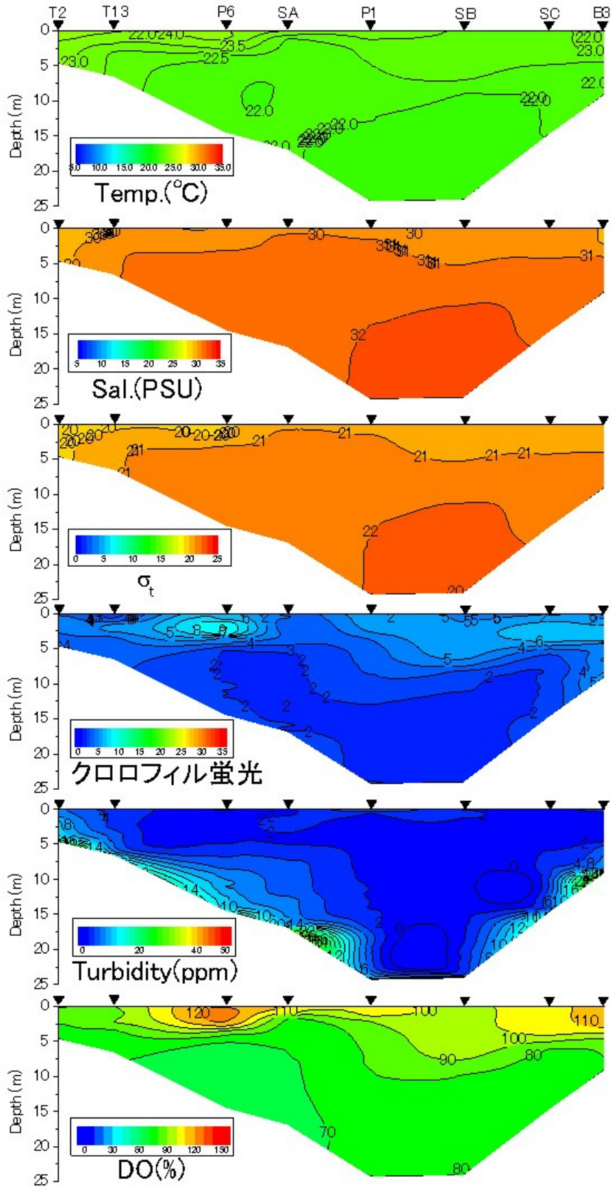
2014年6月29日における水温、塩分、密度 \sigma_t 、クロロフィル蛍光値、濁度、DO飽和度
