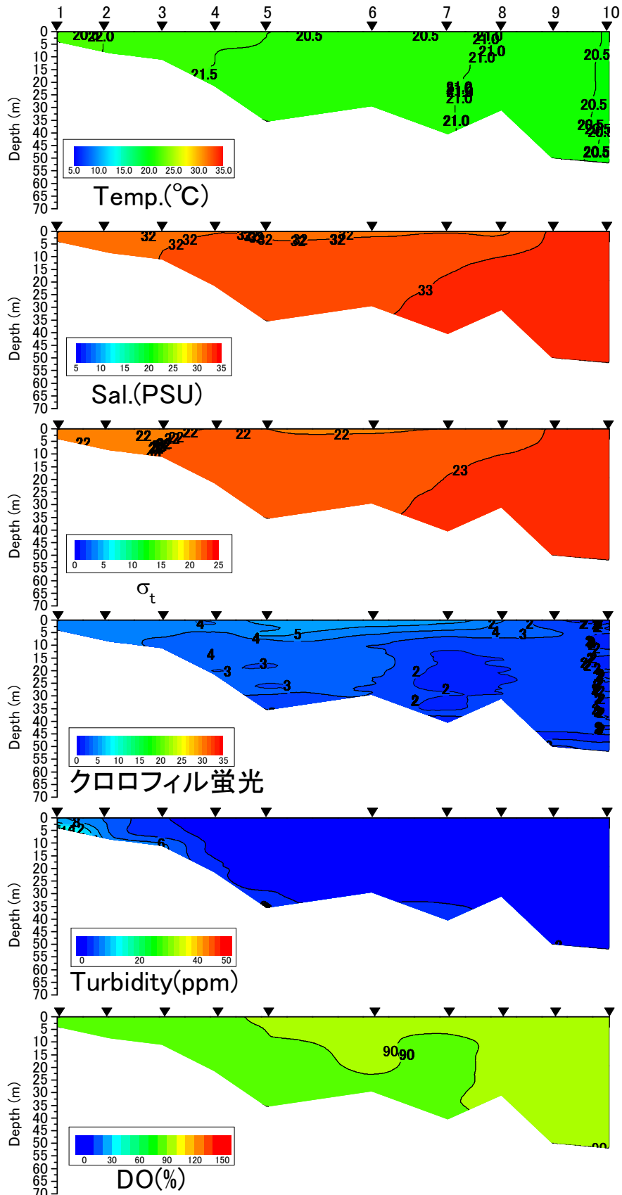
有明海中央ラインの水温(°C)、塩分、密度( \sigma_t )、クロロフィル蛍光強度、濁度、溶存酸素飽和度(DO%)の鉛直面図(国土交通省の調査による) (2014年6月18日)
