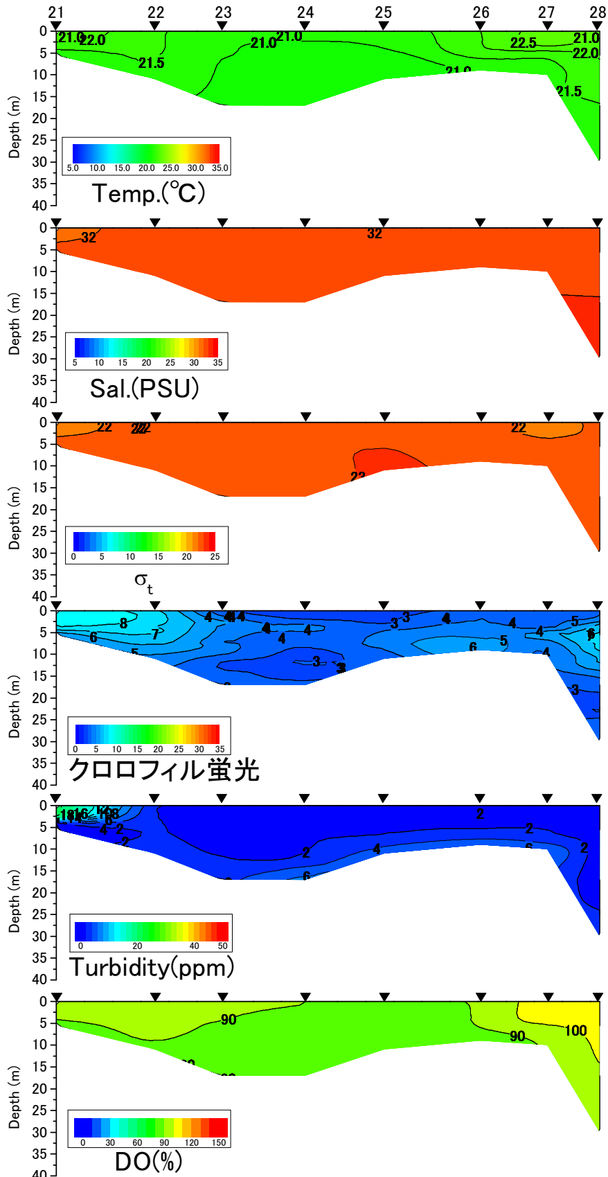
有明海東ラインの水温(°C)、塩分、密度( \sigma_t )、クロロフィル蛍光強度、濁度、溶存酸素飽和度(DO%)の鉛直面図(国土交通省の調査による) (2014年6月12日)
