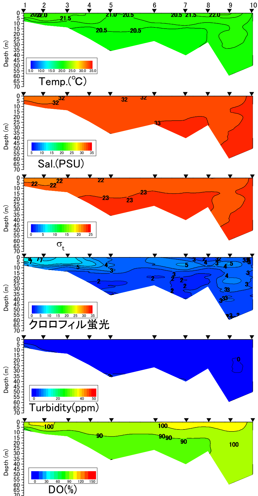
有明海中央ラインの水温(°C)、塩分、密度( \sigma_t )、クロロフィル蛍光強度、濁度、溶存酸素飽和度(DO%)の鉛直面図(国土交通省の調査による) (2014年6月12日)
