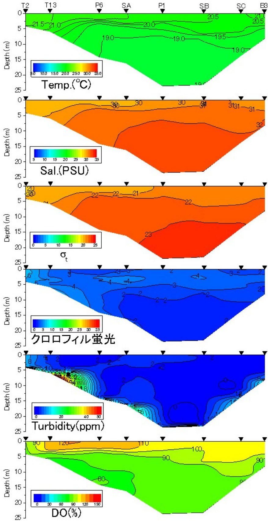
2014年5月25日における水温、塩分、密度 \sigma_t 、クロロフィル蛍光値、濁度、DO飽和度
