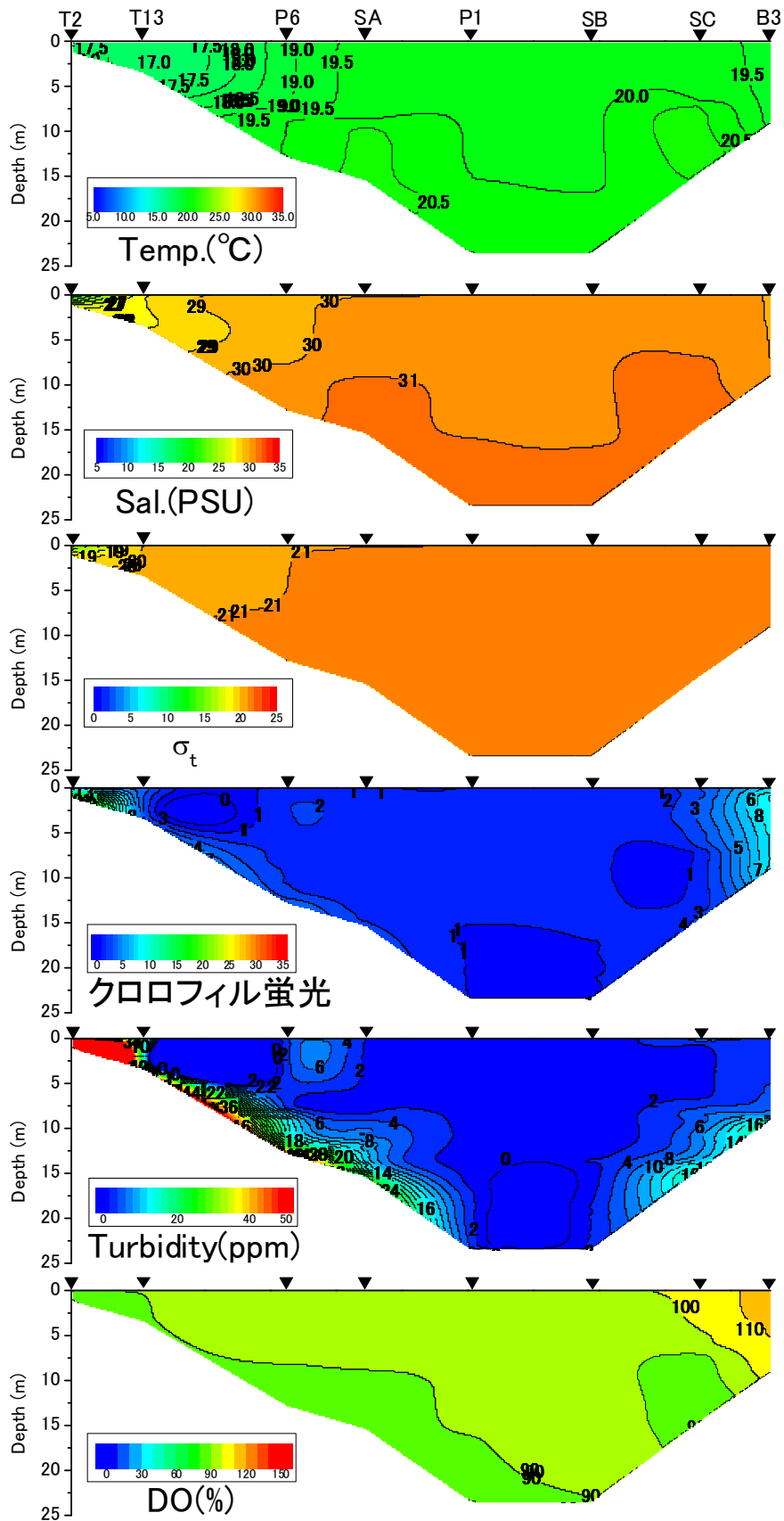
2013年11月11日における水温、塩分、密度 \sigma_t 、クロロフィル蛍光値、濁度、DO飽和度
