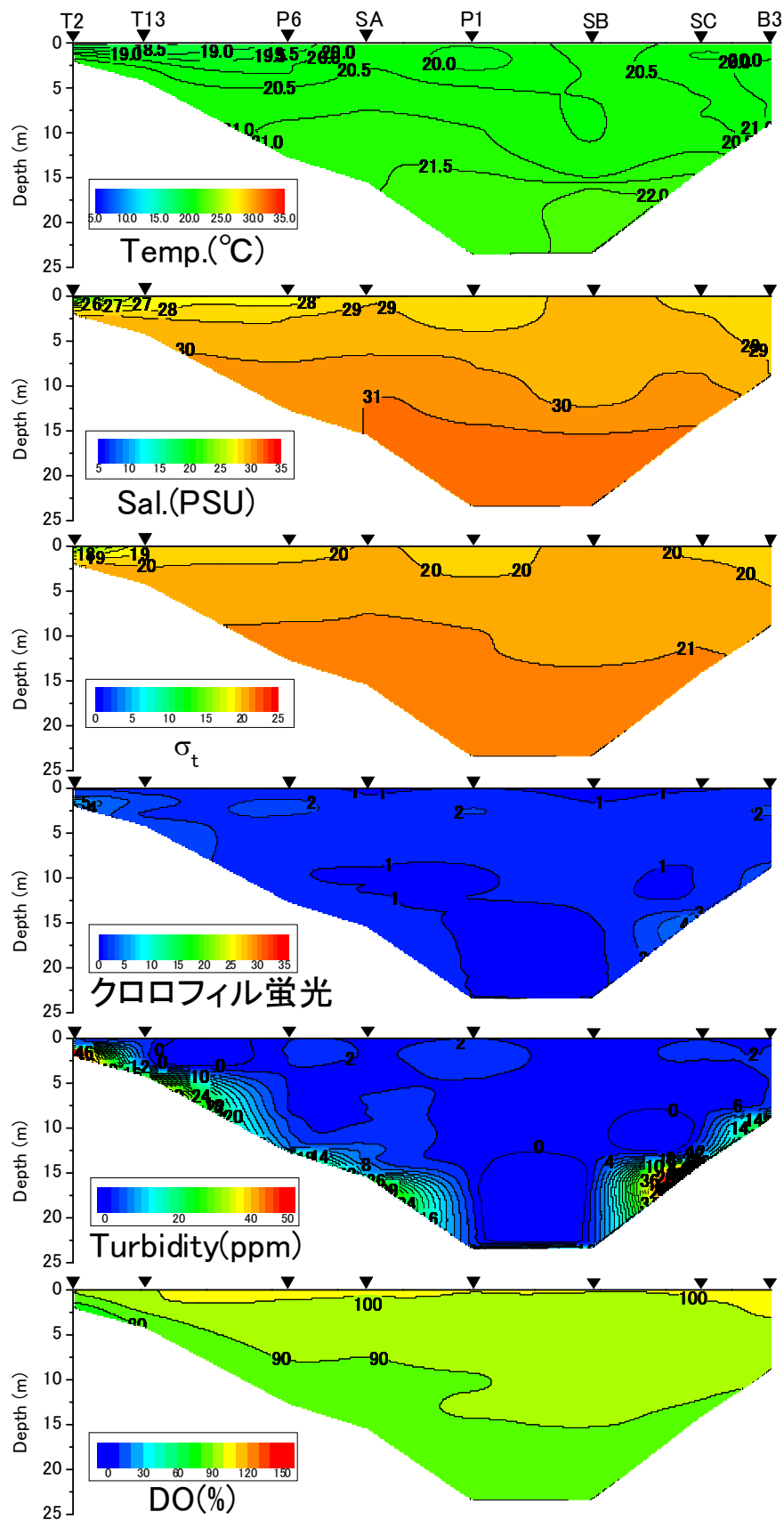
2013年10月27日における水温、塩分、密度 \sigma_t 、クロロフィル蛍光値、濁度、DO飽和度
