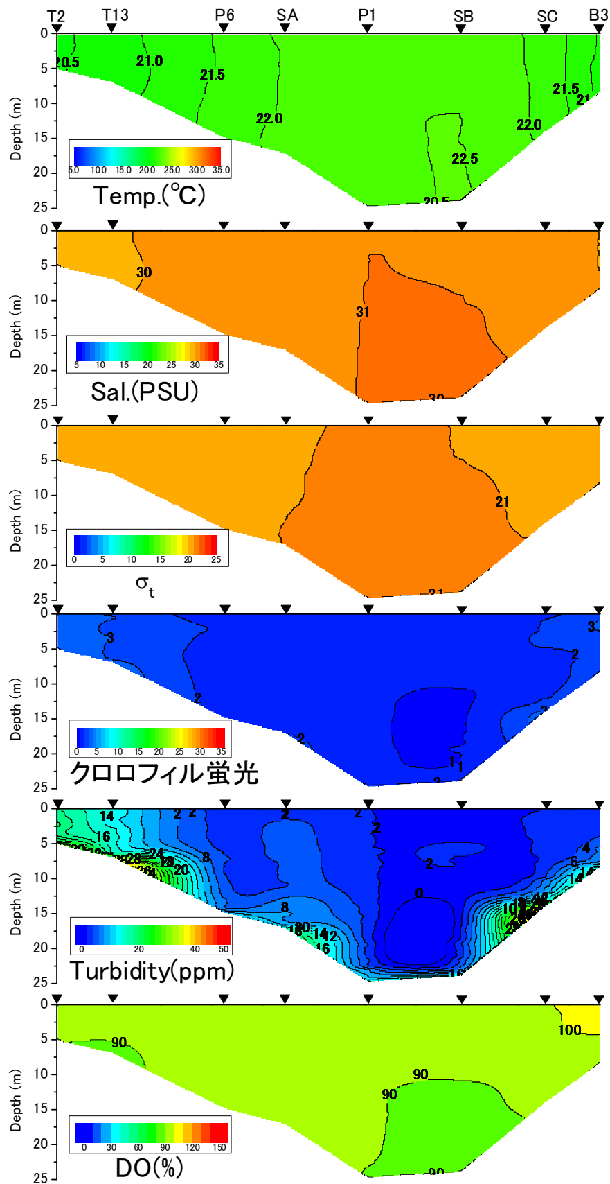
2013年10月20日における水温、塩分、密度 \sigma_t 、クロロフィル蛍光値、濁度、DO飽和度
