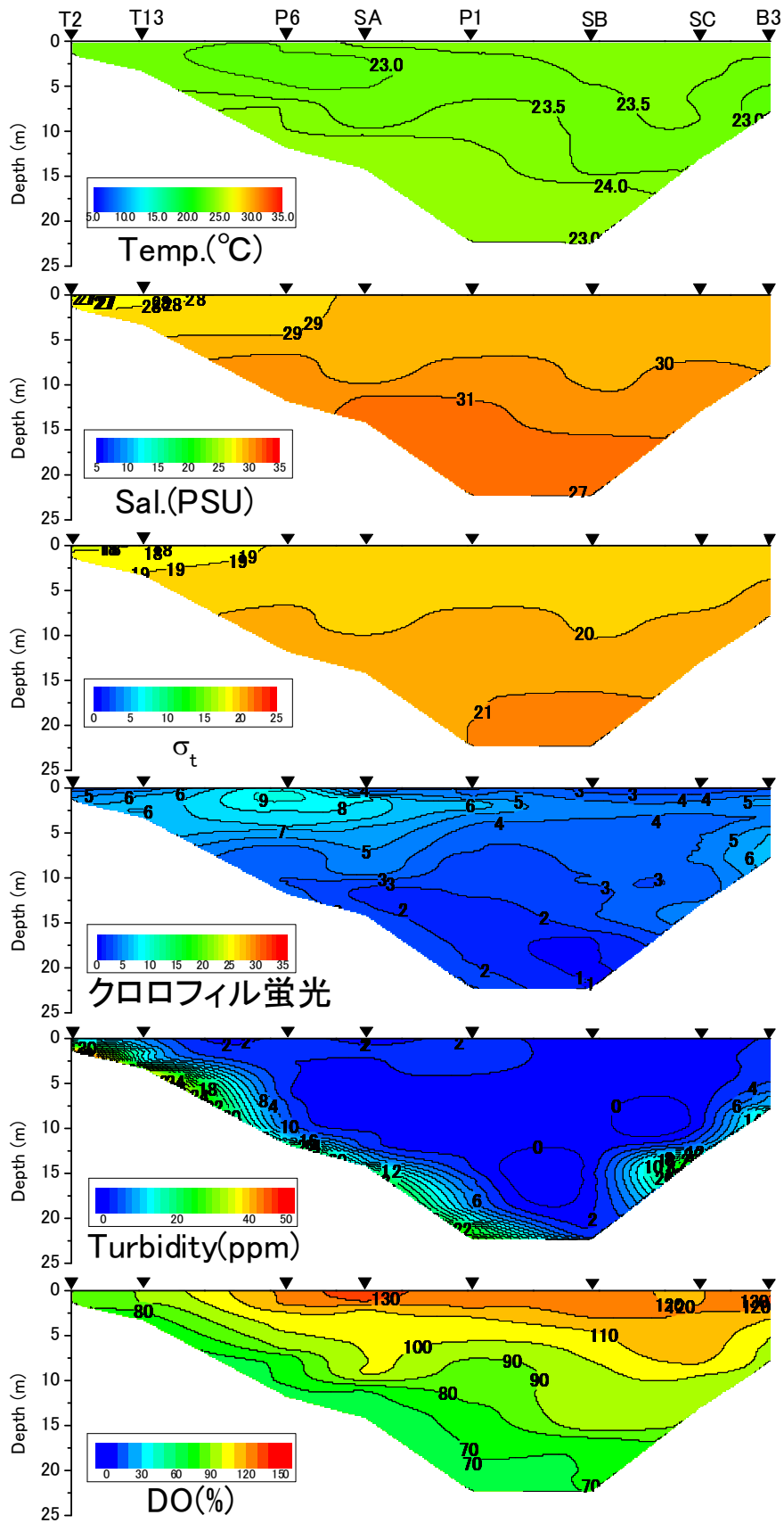
2013年10月14日における水温、塩分、密度 \sigma_t 、クロロフィル蛍光値、濁度、DO飽和度
