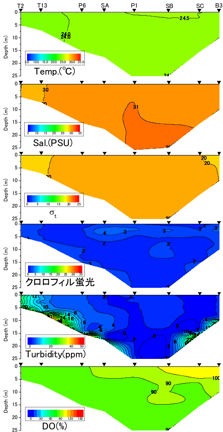
2013年10月7日における水温、塩分、密度 \sigma_t 、クロロフィル蛍光値、濁度、DO飽和度
